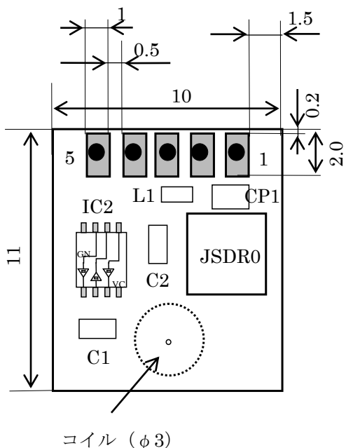
<部品実装面>
