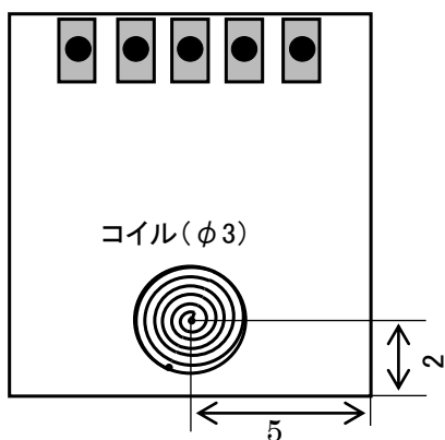
<部品実装面>
