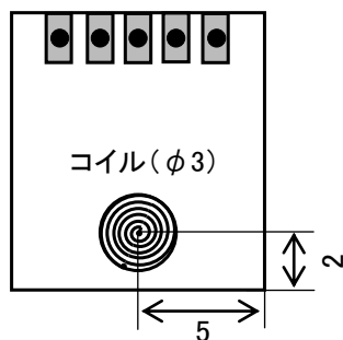
<部品実装面>
