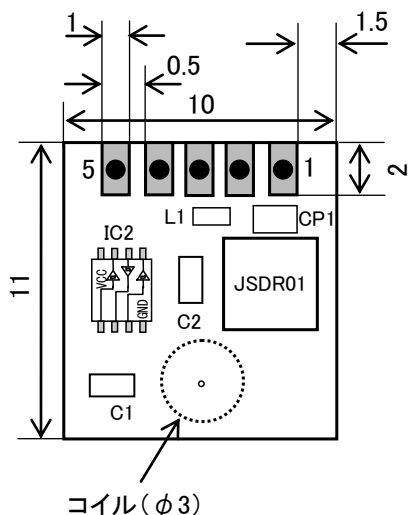
<部品実装面>
